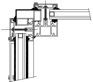
TYMPAN
