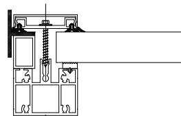
COTE OUVERT
